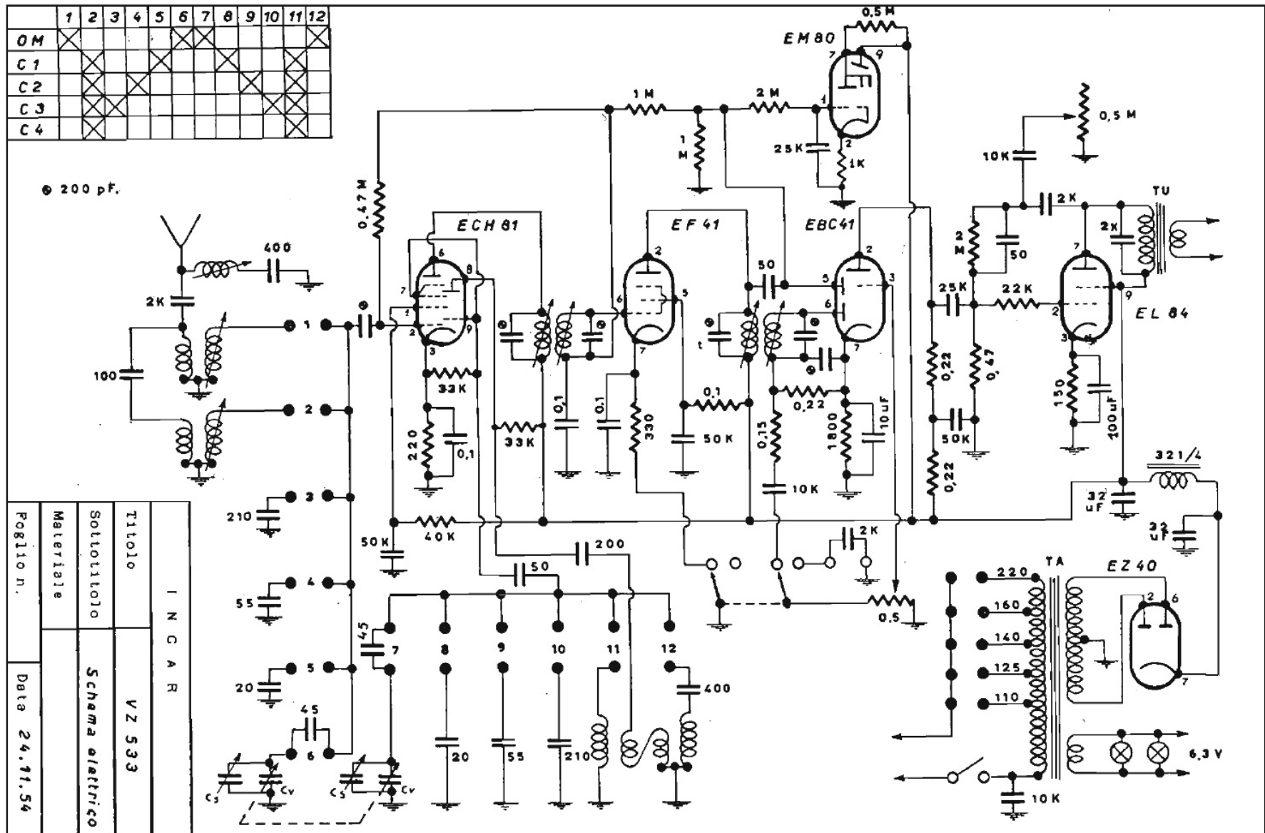
INCAR - Mod. VZ 533. Ricevitore a onde medie con quattro bande allargate in onde corte. Potenza d'uscita 3 watt. Consumo 50 watt.
